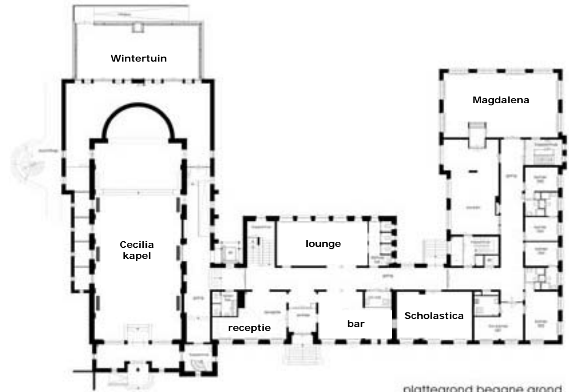
plattegrond begane grond overzicht
